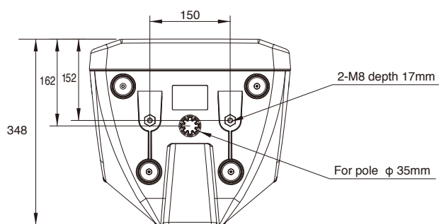
底面図
