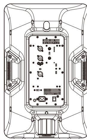
背面図
